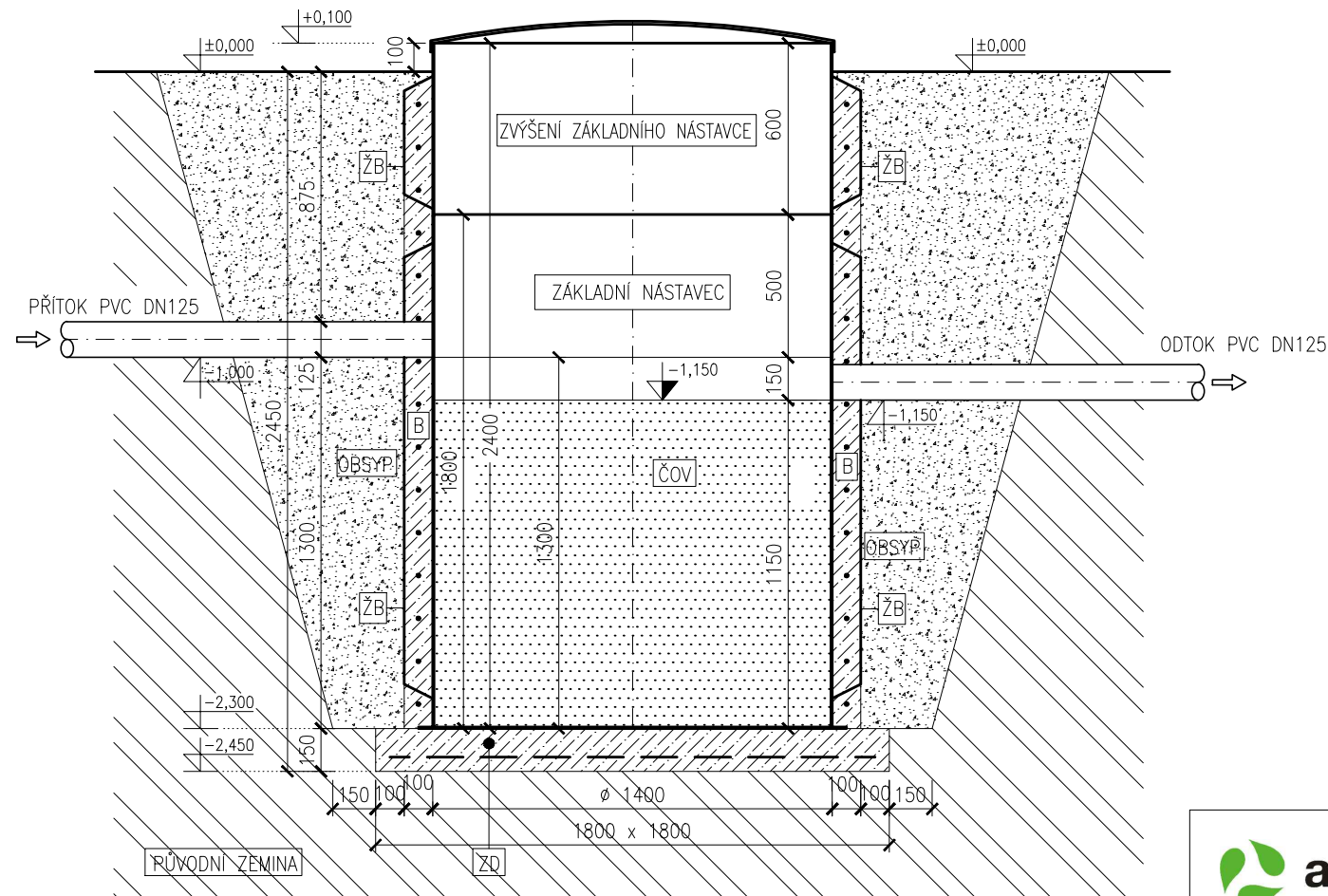
Řez
