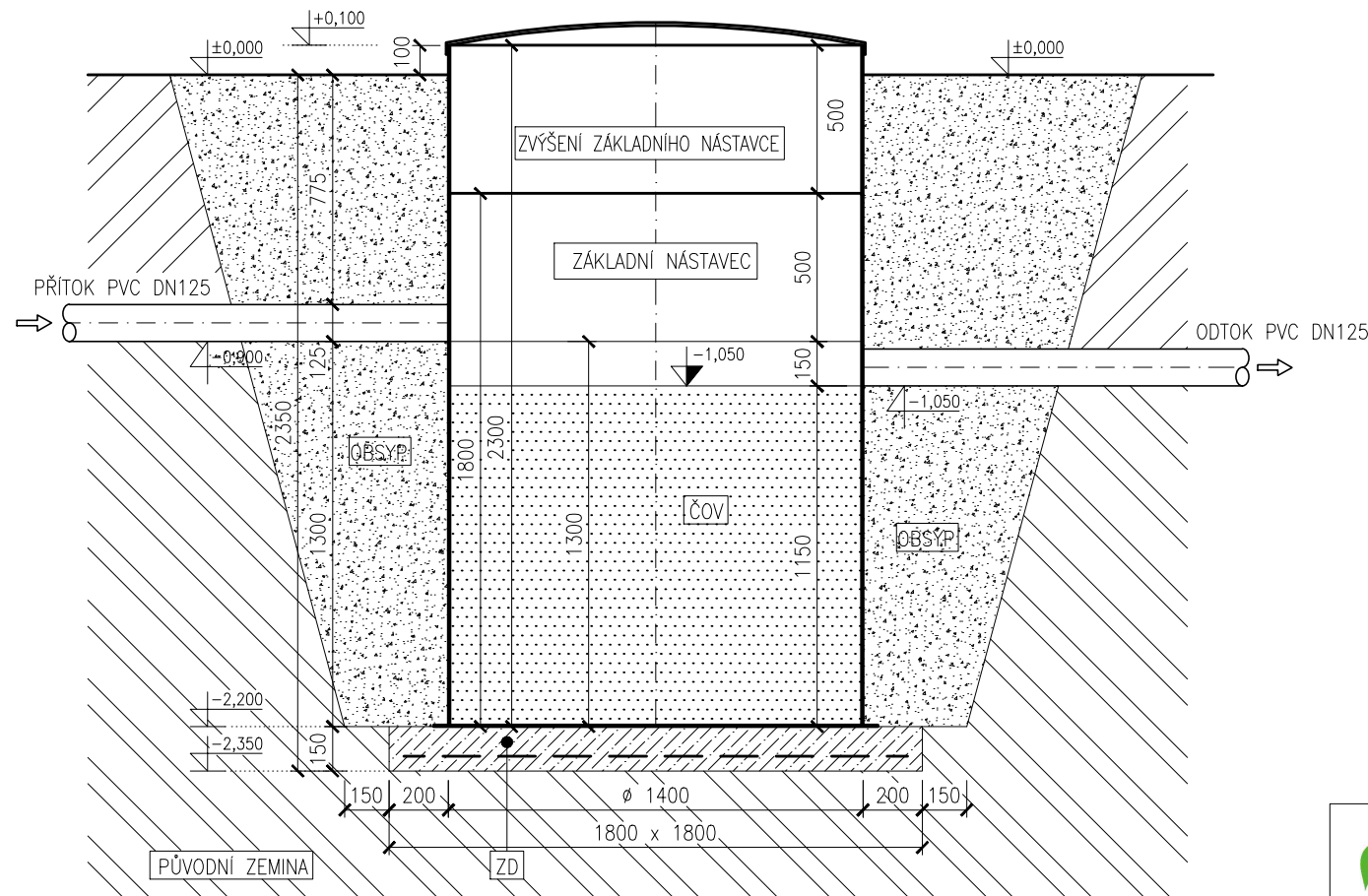
Řez
